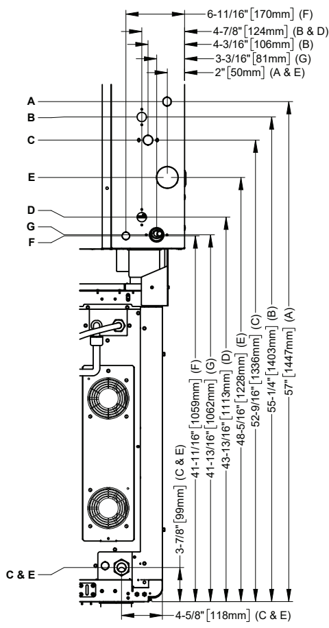
DETAIL Y
